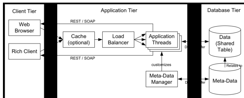
Abbildung 1: Mehrmandanten-Architekturstil SPOSAD, aus Koziolk [Ko10]
