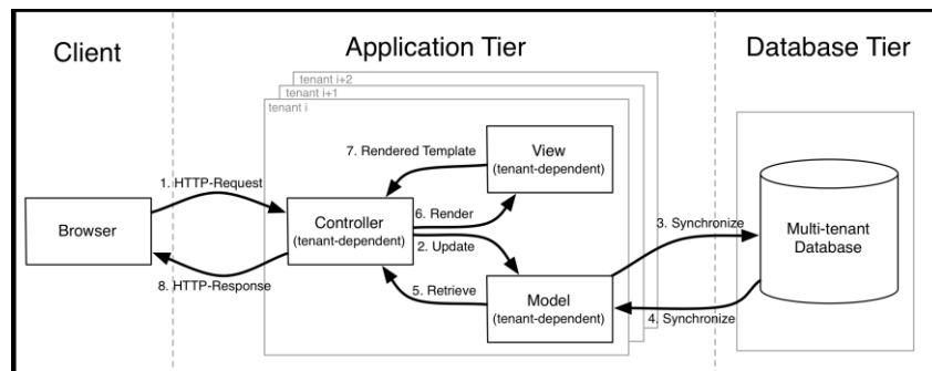
Abbildung 2: Mehrmandanten-Architektur von Hallway im Play!-Framework
