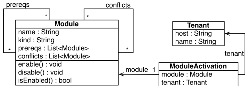
Abbildung 3: Modul-System zum Austausch unterschiedlicher zu untersuchender Mechanismen
